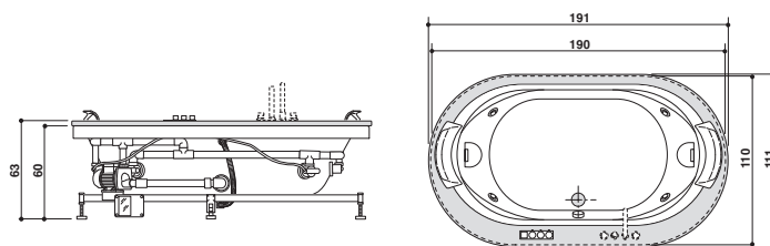
Asiento doble · Два сиденья
