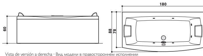
Vista de versión a derecha · Вид модели в правостороннем исполнении
