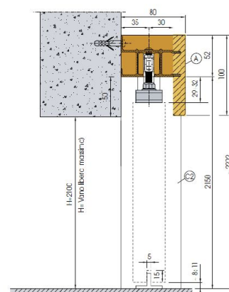
Sezione verticale
