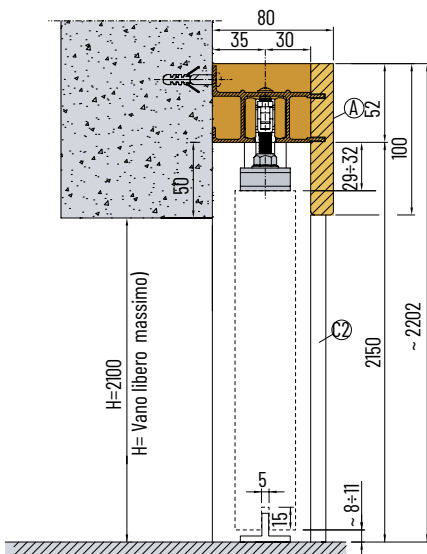
Sezione verticale
