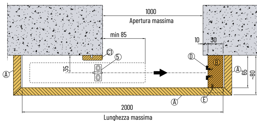
Sezione orizzontale
