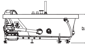
Left hand version view · Abb. Linksausführung
