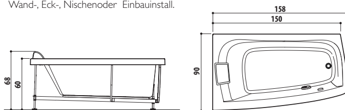
Left hand version view · Abb. Linksausführung
