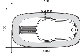
Left hand version view · Abb. Linksau sführung
