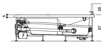
Left hand version view · Abb. Linksausführung
