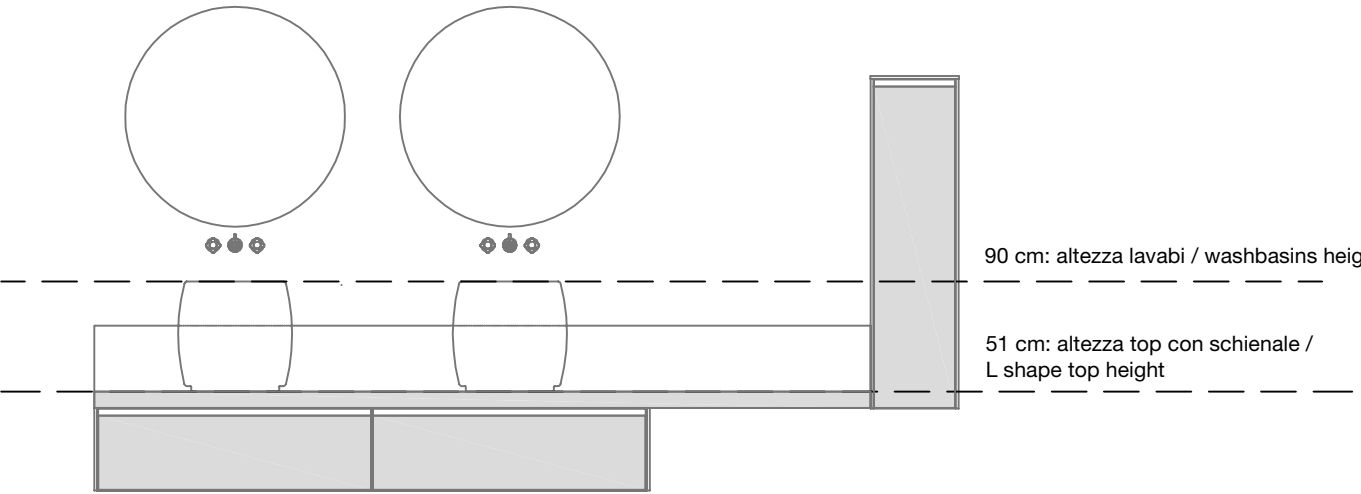
BASI H30 CON TOP CON SCHIENALE E LAVABI IN APPOGGIO CABINETS H30 WITH L SHAPE TOP AND COUNTERTOP WASHBASINS
