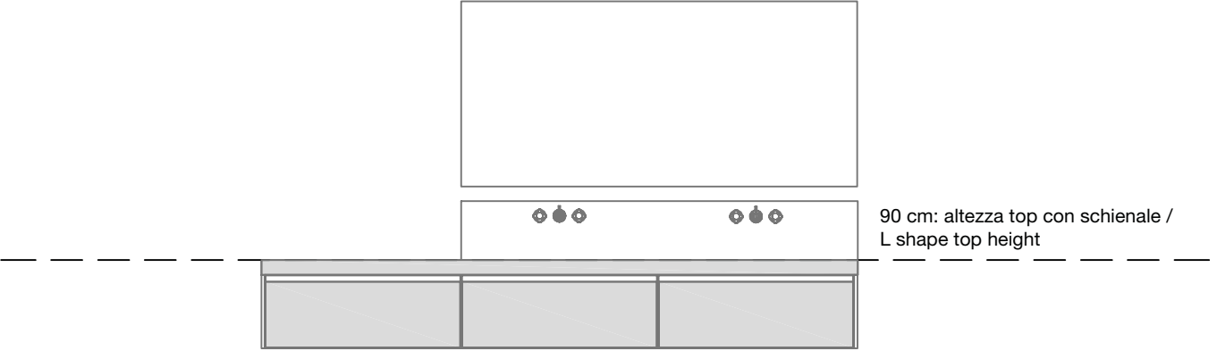
BASI H30 CON TOP CON SCHIENALE E LAVABO INTEGRATO CABINETS H30 WITH L SHAPE TOP AND INTEGRATED WASHBASIN
