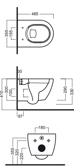
vaso sospeso PURE RIM PURE RIM wall hung wc
