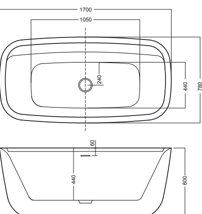
vasca 170x78 BT_03 bathtub 170x78 BT_03
