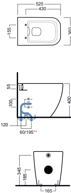
vaso filo muro PURE RIM_SCARICO TRASLATO PURE RIM back to wall wc_SHIFT DRAIN SYSTEM
